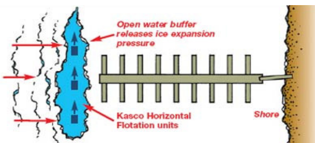
Isfri bufferzone ved hjælp af flydeenhed
